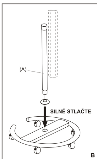
B Nasadte spojovací víčko na trubku "A" a připojte ke kruhové základně.
